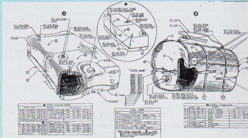
Nákres zachycující řešení samosvorných nádrží
