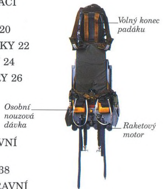
MODERNÍ VYSTŘELOVACÍ SEDADLO
