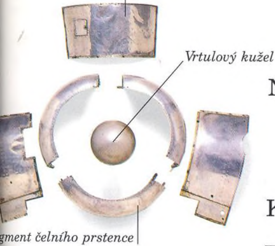
MOTOROVÝ KRYT LETOUNU LOCKHEED ELECTRA, 1934
