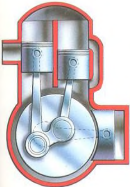
Řez dvouválcovým motorem
