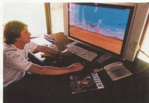
DVACETIKILOMETROVÝ ASTEROID
