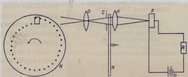
Obr. 3. Nipkovův kotouč a jeho použití ve vysílači.
