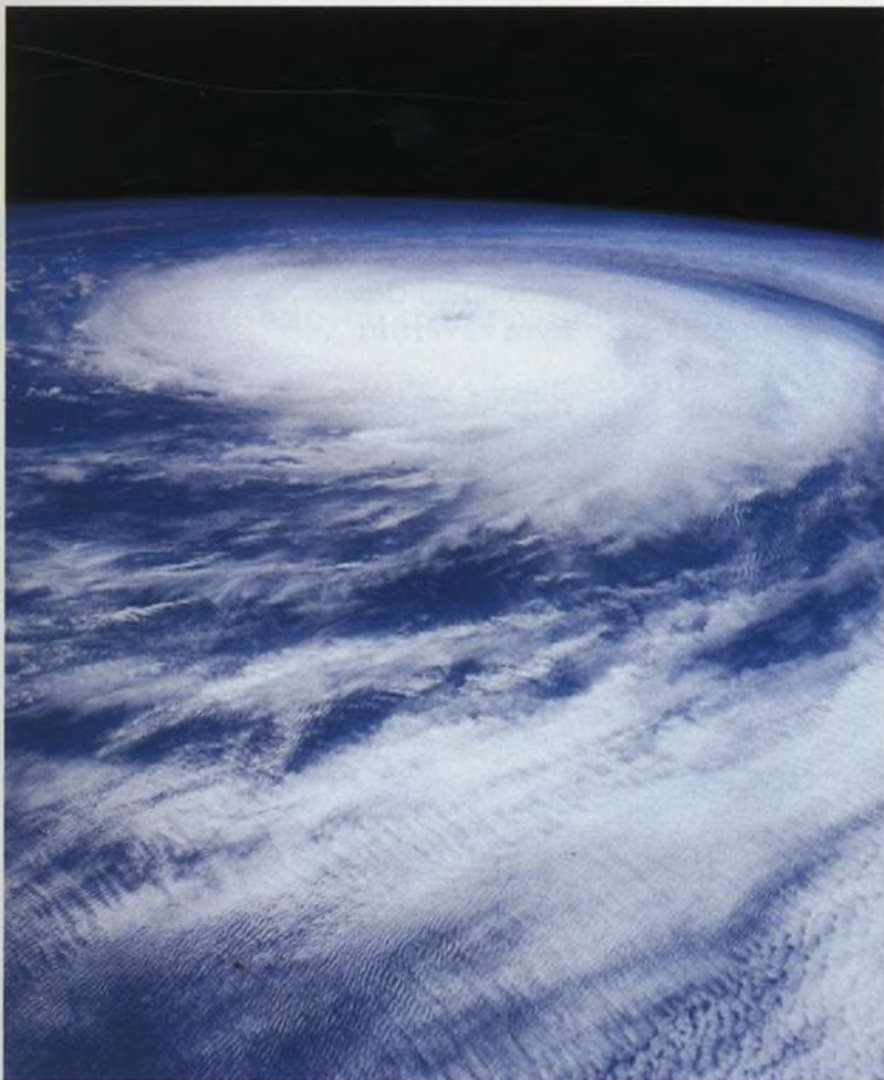
Hurikán Feba nad Tichým oceánem v srpnu 1991
