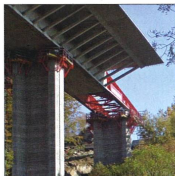
Dálniční most přes údolí Rybného potoka
